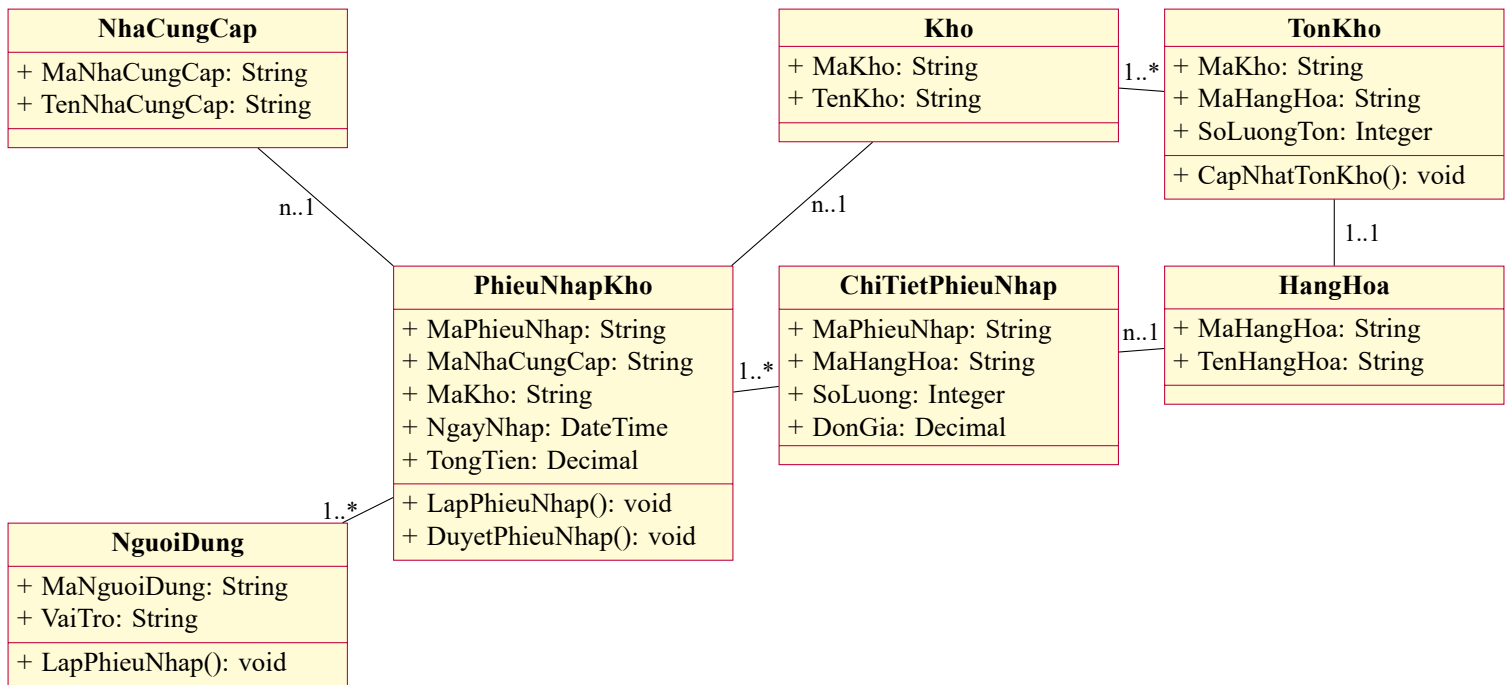
Hình 1: Biểu đồ lớp trong ca sử dụng UC09 – Lập phiếu nhập kho
